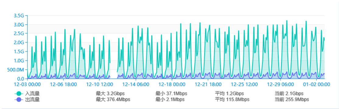
图 9 为移动代拨出口流量详情，其中最大入流量 3.2Gbps,平均入流量 1.2Gbps，出流量最大 376.4 Mbps，平均出流量 115.8Mbps
