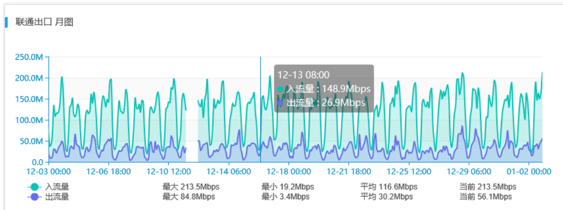
图 2 为本月联通出口流量详情，其中最大入流量 213.5Mbps,平均入流量 116.6Mbps，出流量最大 84.8Mbps，平均出流量 30.2Mbps。
