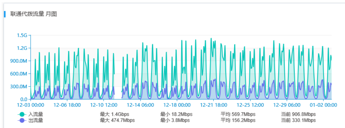
图 8 为联通代拨出口流量详情，最大入流量 1.4 Gbps,平均入流量 569.7Mbps，出流量最大 474.7 Mbps，平均出流量 156.2 Mbps。
