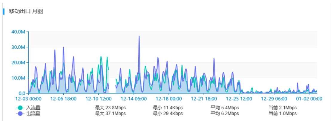
图 3 为移动出口流量详情，其中最大入流量 23.8Mbps,平均入流量 5.4Mbps，出流量最大 37.1Mbps，平均出流量 6.2Mbps。由于移动线路近段时间内在做线路改造，导致其网络质量不佳，故使用人数较少。
